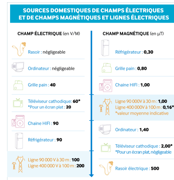
Figure 202 : Exemple de champs magnétiques et électrique (Source : RTE France)
